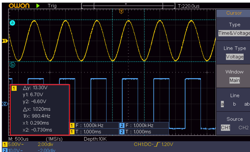
Figure 4-15 Time&Voltage カーソル測定
