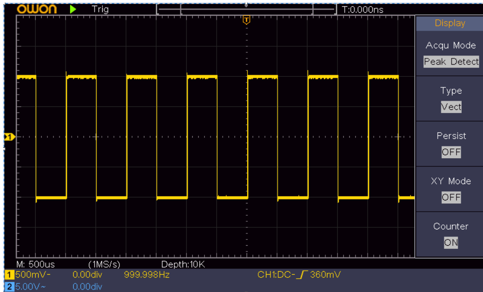
Figure 6-4 ノイズを含む信号
