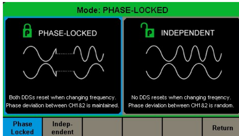
図 82 モード設定インターフェース
