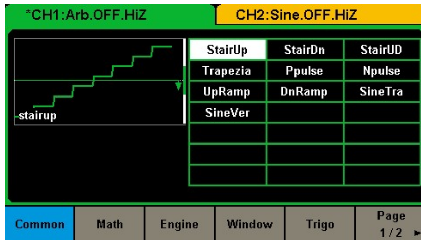
21 内蔵任意波形
