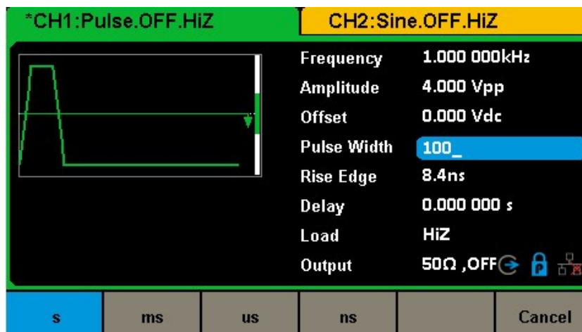
図 11 パルス幅の設定
