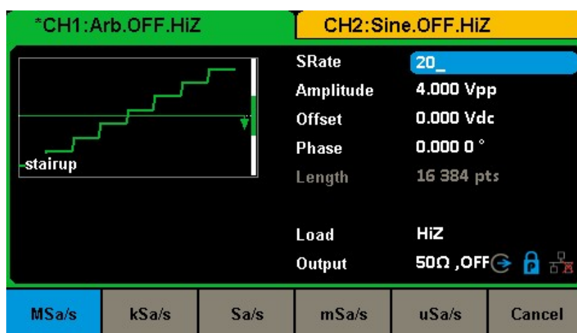
図 20 サンプリングレートの設定
