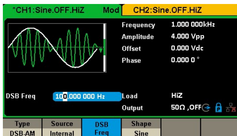
図 25DSB-AM 変調の 設定インターフェース
