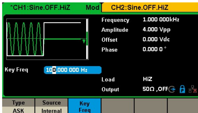
図 29 ASK 変調設定インターフェース
