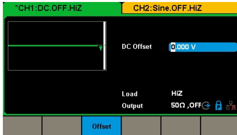
図 17DC 設定インターフェース
