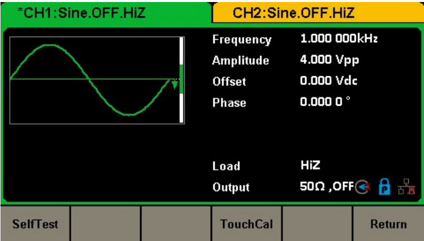
図 59 テスト/校正機能メニュー
