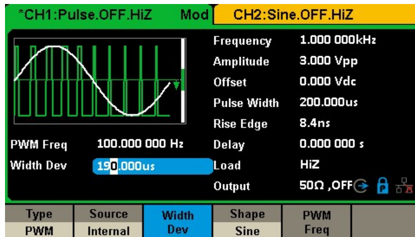
32 幅偏差設定インターフェース
