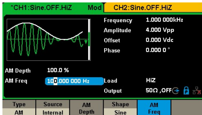
図 24 AM 変調設定インターフェース
