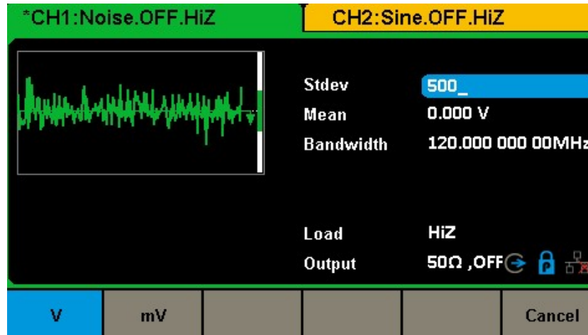
図 14 Stdev の設定
