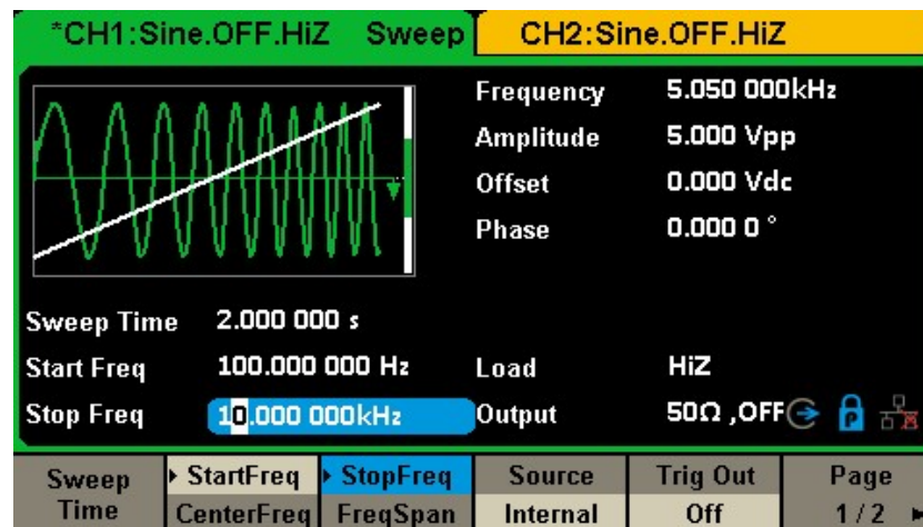
図 7 による直線掃引波形の生成
