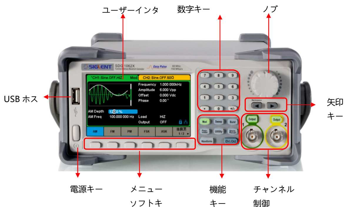
図 2SDG2000X のフロントパネル
