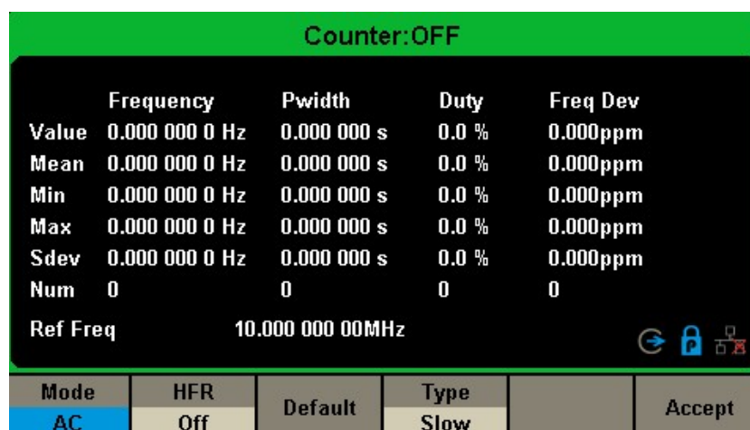
図 68 カウンタ設定インターフェイス
