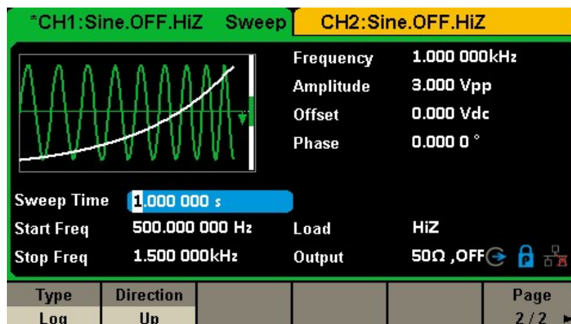
図 37 対数スイープインターフェース
