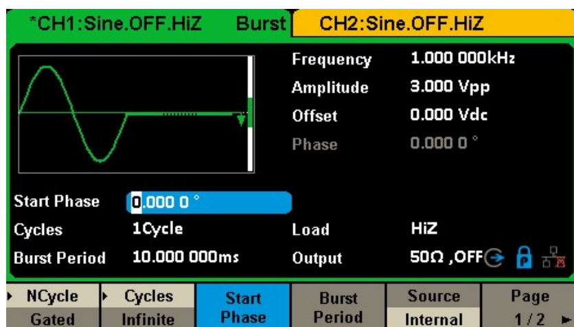
図 -238 N サイクルバーストインターフェース (1/2 ページ)
