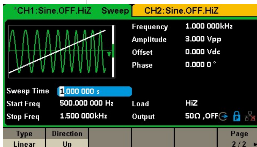
図 35 スイープの設定インターフェース (2/2 ページ)
