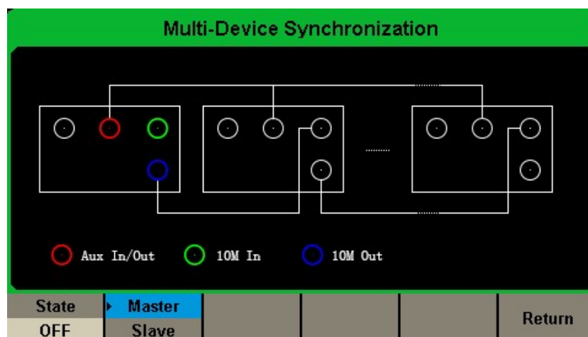
図 86 マルチデバイス同期インターフェース
