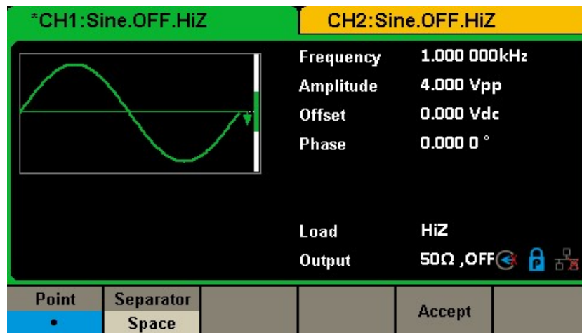
図 254 数値形式の設定
