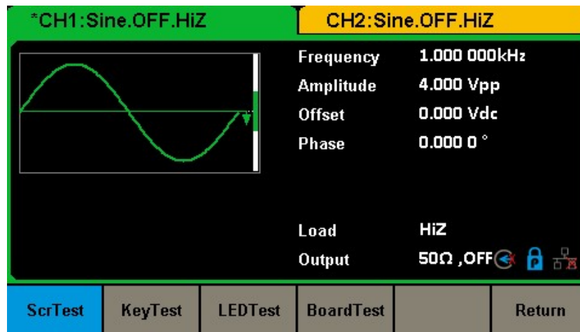
図 60 セルフテストインターフェース
