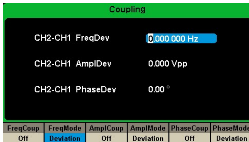
図 273 チャンネル結合インターフェース
