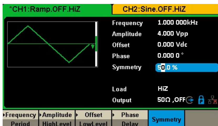
8 ランプ波形パラメータ表示インターフェース
