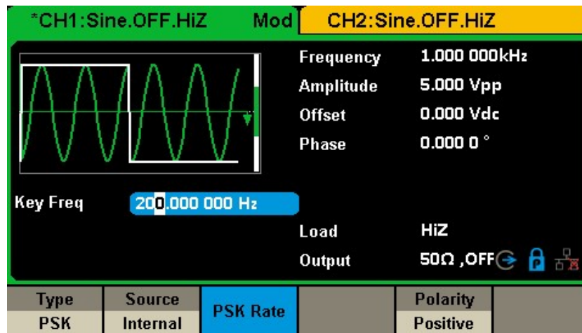
図 14 PSK 変調波形を生成
