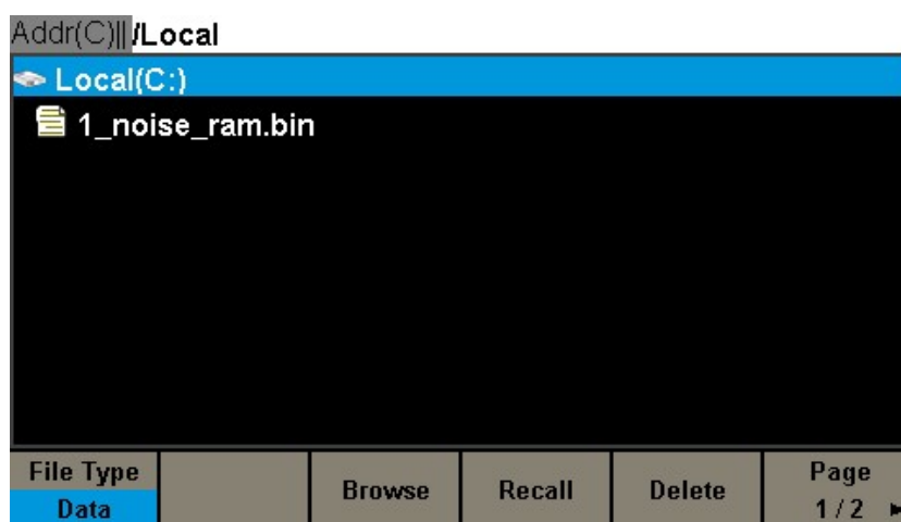
図 22 保存波形表示インターフェース
