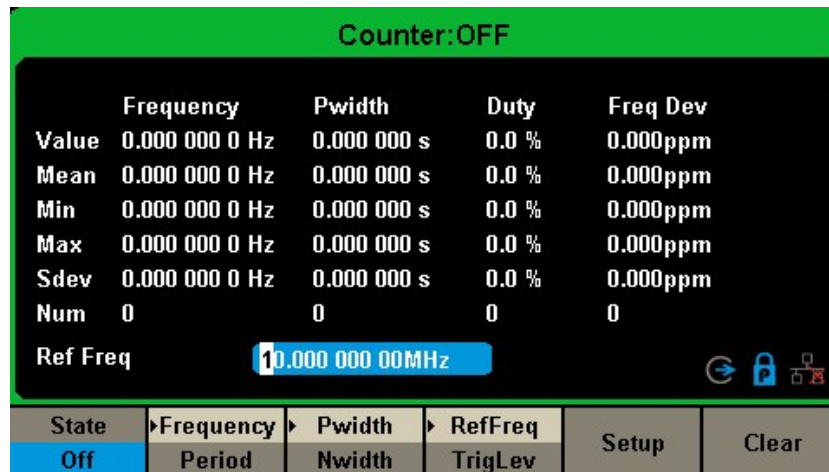
図 67 周波数カウンタインターフェース
