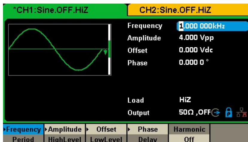
図 83 位相ロックモード
