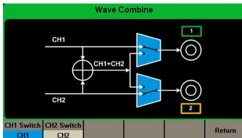
図 71 波形結合インターフェース
