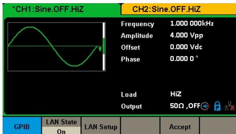
図 78 インターフェース設定
