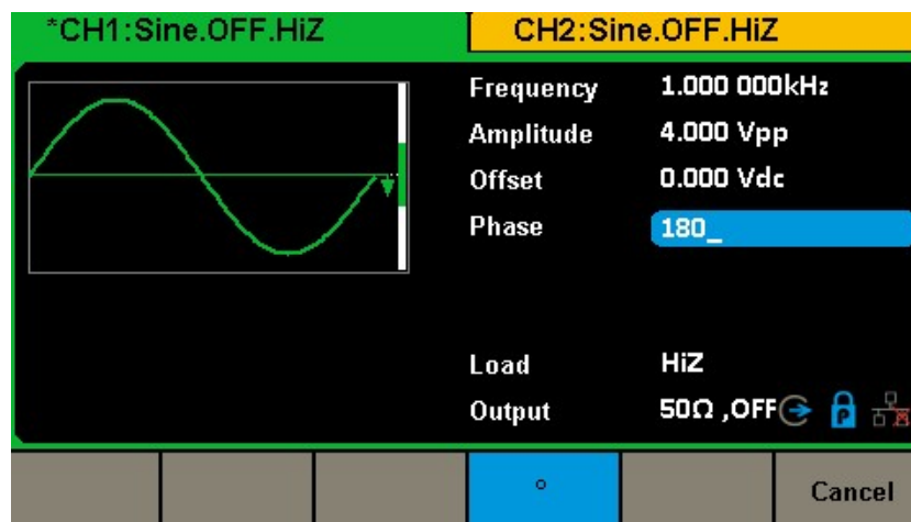
図 5 位相の設定
