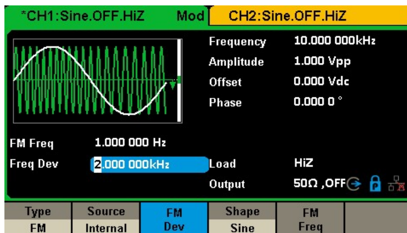
図 10 による FM 変調波形の生成
