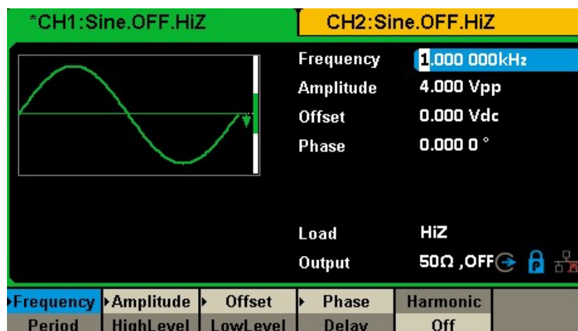
図 6 正弦波表示インターフェース
