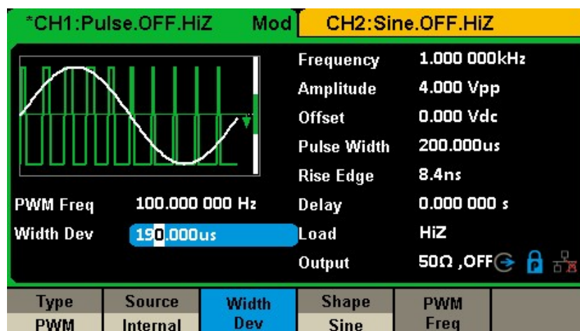
図 31PWM 変調の 設定インターフェース
