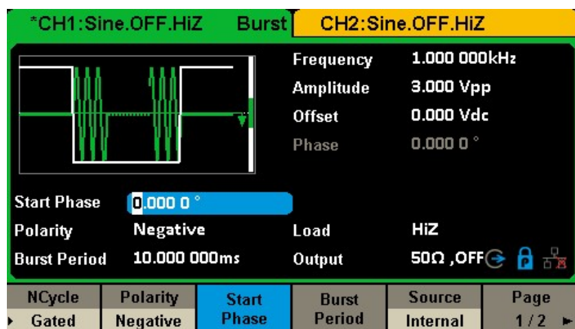
図 41 ゲート付きバーストインターフェイス (1/2 ページ)
