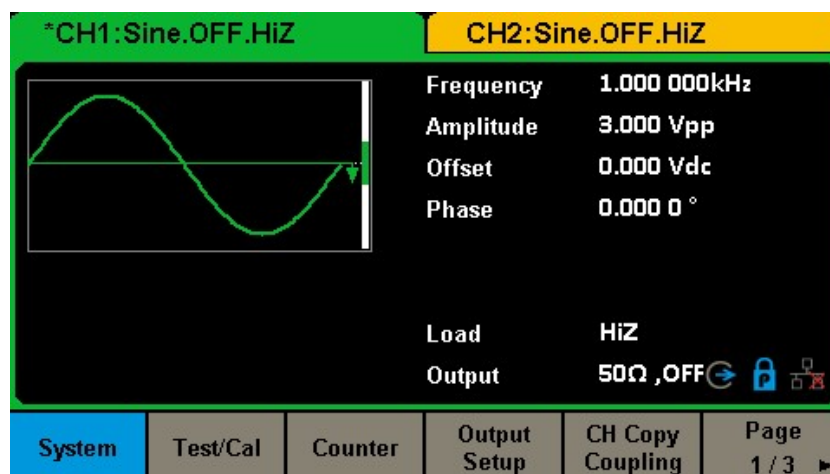
図 47 ユーティリティ設定インターフェイス (1/3 ページ)
