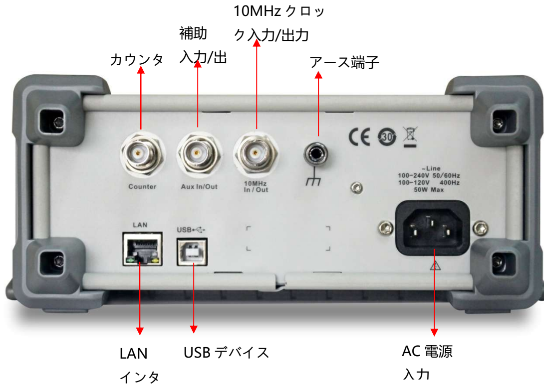
図 3SDG2000X の背面パネル
