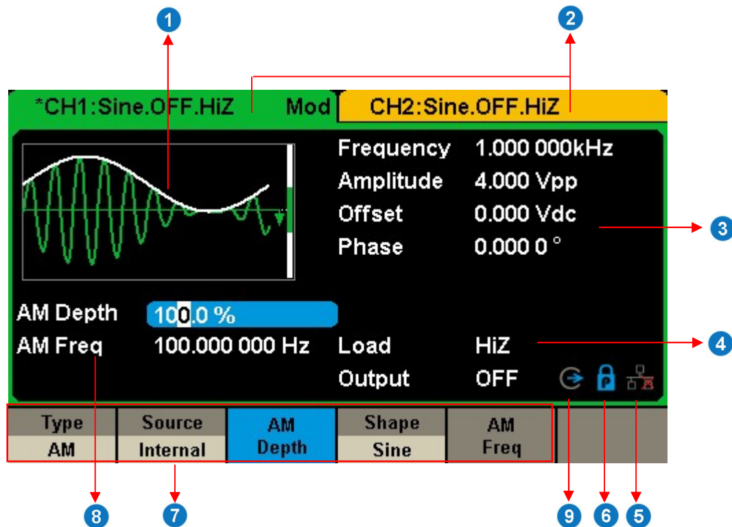
図 14 タッチスクリーン表示
