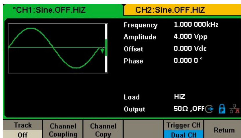
図 77 チャンネルトリガー信号の相関
