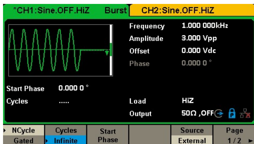
図 40 無制限バーストインターフェイス
