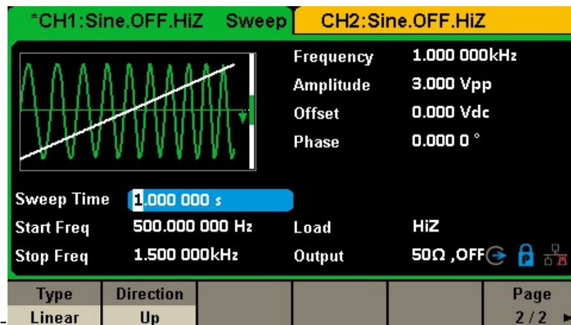
図 36 リニアスイープインターフェース
