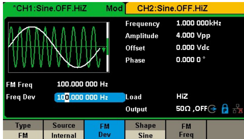
26 FM 変調設定インターフェース
