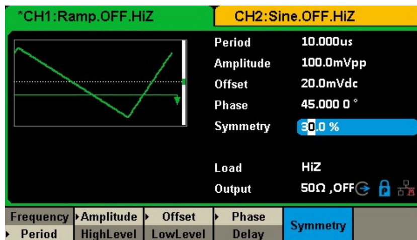
図 3 ランプ波形を生成
