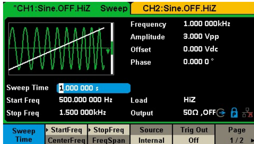
図 34 スイープ設定インターフェース (1/2 ページ)
