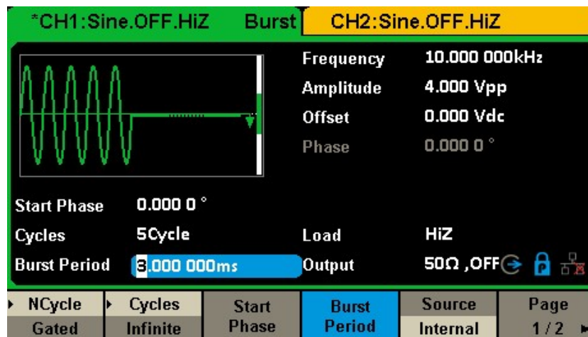
図 8 N サイクルバースト波形を生成する
