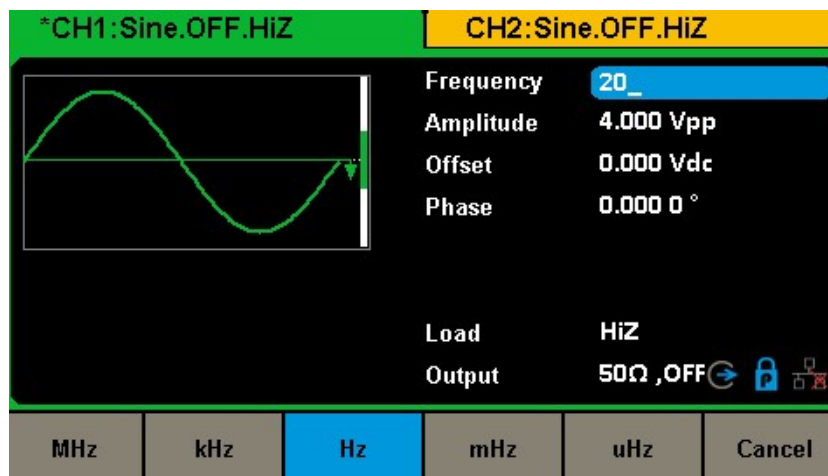
2 周波数の設定
