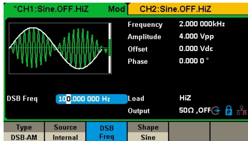
図 16 DSB-AM 変調波形を生成
