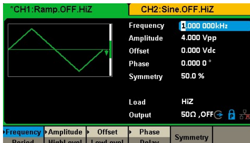
図8 ランプ表示インターフェース
