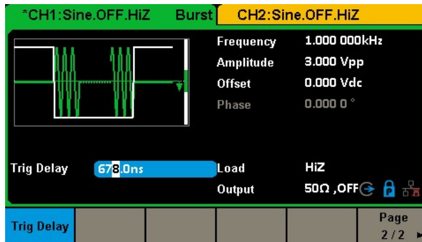
図 42 ゲート付きバーストインターフェース (2/2 ページ)
