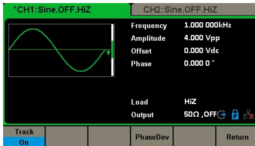
図 74 トラックインターフェース
