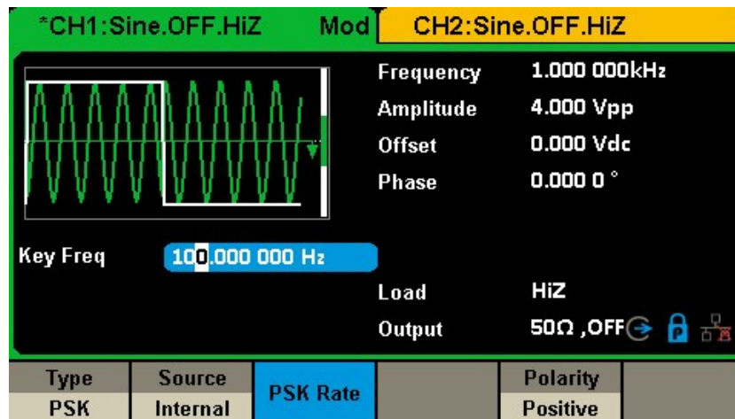
図 30 PSK 変調の設定インターフェース
