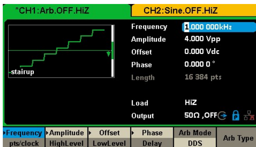
図 18 任意波形パラメータ表示インターフェース (DDS)
