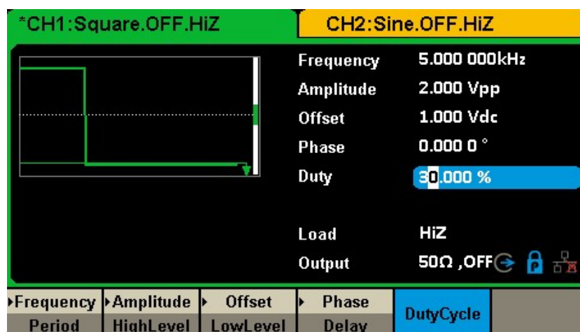
図 2 矩形波の生成
