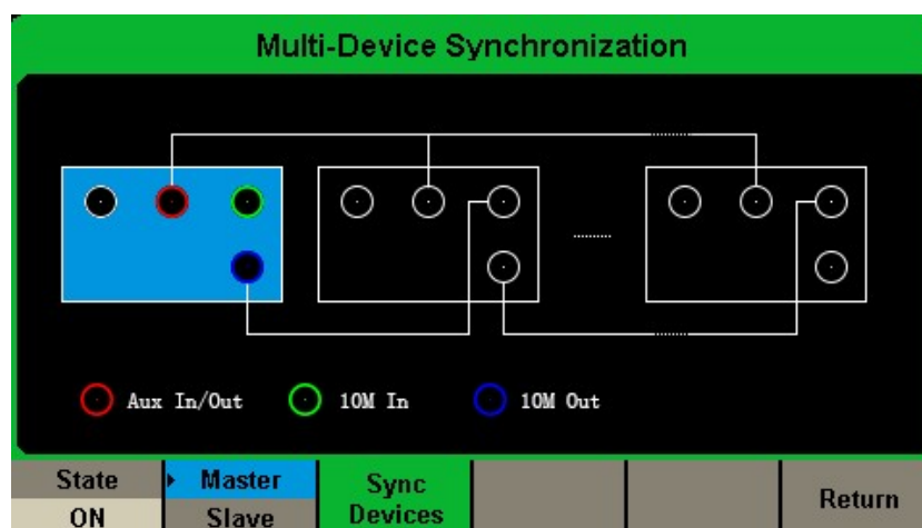
87 マスターモードインターフェース
