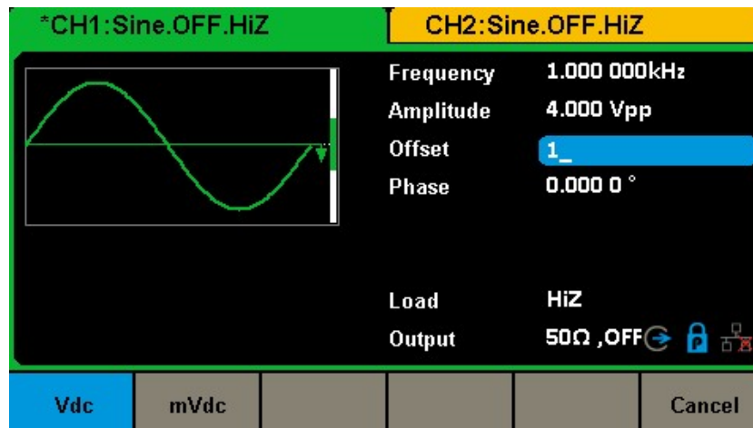
図 4 オフセットの設定
