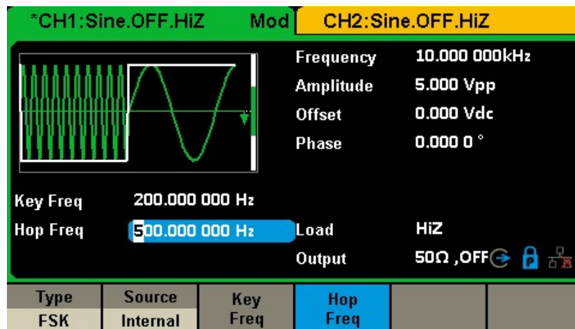
図 12 による FSK 変調波形の生成
