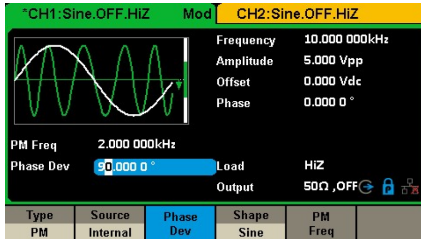
図 11 による PM 変調波形の生成
