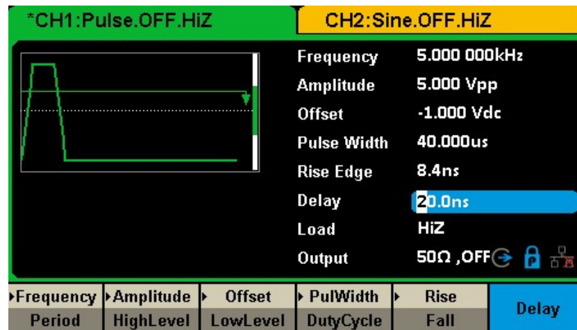
図 4 パルス波形を生成する
